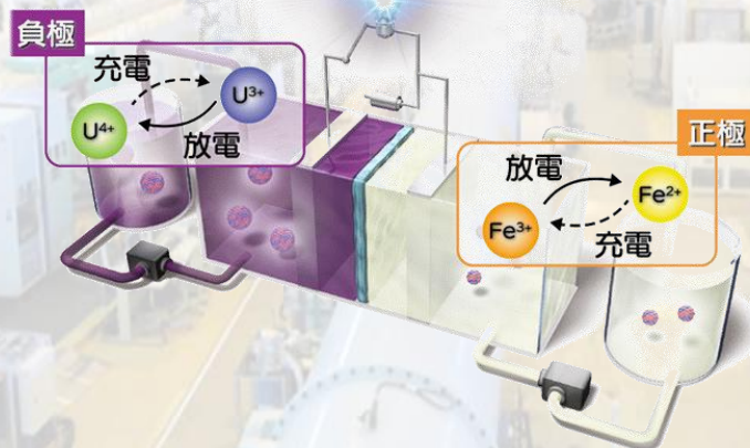
ウランレドックスフロー蓄電池
