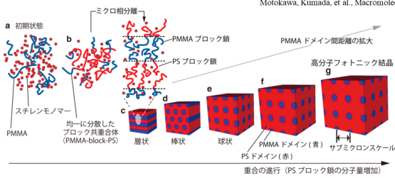
図. ブロック共重合体の重合誘起相分離を利用した高分子フォトニック結晶作製スキーム。
