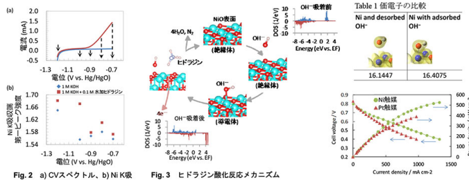
Fig. 2 a) CVスペクトル, b) Ni K吸収第一ピーク強度と電位との関係
