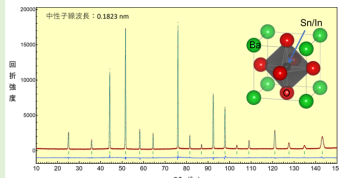
図1 水素伝導体BaSn 0.5 In 0.5 O 2.75 のリートベルト解析
