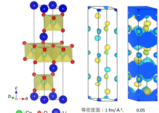
図3 リチウムイオン二次電池正極材の結晶構造と原子核密度
