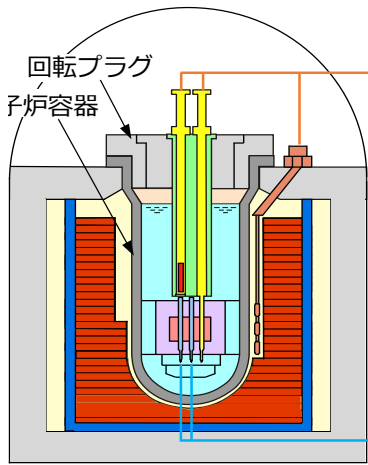
「常陽」の照射場
