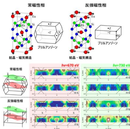
(図1) EuRh2Si2の磁気構造と、ARPESによって実験的に決定したフェルミ面の温度変化。反強磁性転移によってブリルアンゾーンが折りたたまれる様子が観測されている。
