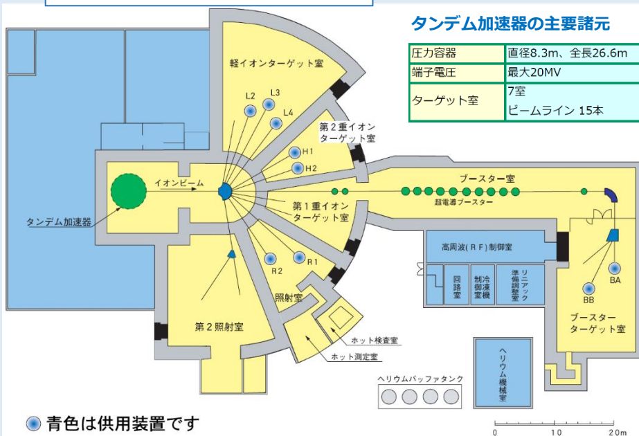
タンデム加速器施設の機器配置図
