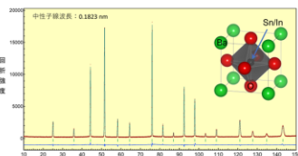
図1 水素伝導体 \text{BaSn}_{0.5}\text{In}_{0.5}\text{O}_{2.75} のリートベルト解析
