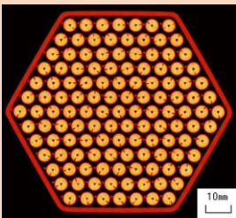
炉心燃料集合体の断面像
