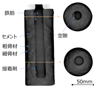
図1 鉄筋コンクリート内部の様子
