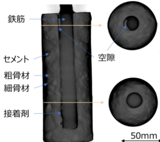
図1 鉄筋コンクリート内部の様子
