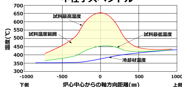
材料照射の場合の試料温度(第6列)
