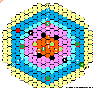
「常陽」の照射場
