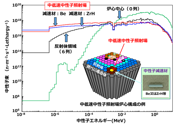
中性子スペクトル
