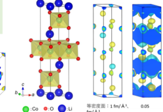
図3 リチウムイオン二次電池正極材の結晶構造と原子核密度
