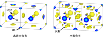
図2 BaSn 0.5 In 0.5 O 2.75 の原子核密度分布図(単位胞を2つ並べて表示)
