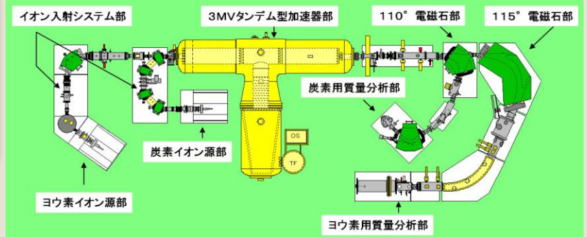
タンデトロン配置図
