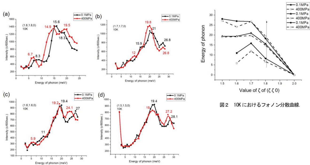
図1 10Kにおける非弾性散乱の \omega スキャン. (a)-(d)はそれぞれ \zeta=1.8, 1.7, 1.6, 1.5 .
