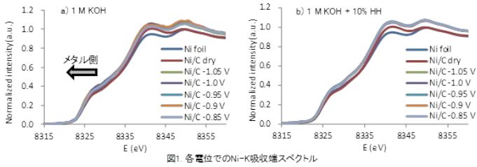
図1. 各電位でのNi-K吸収端スペクトル
