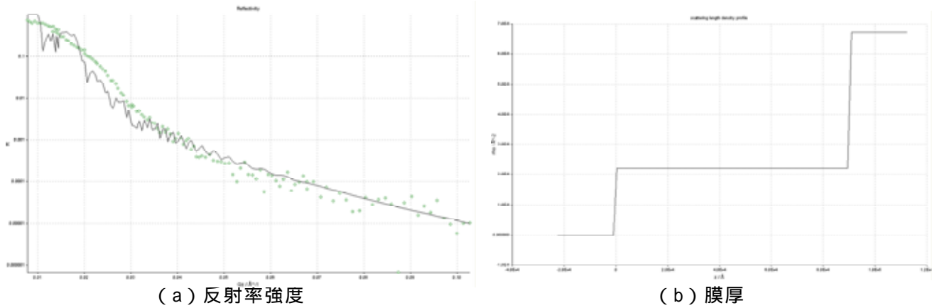
図 5 TRD 処理の VC 皮膜
