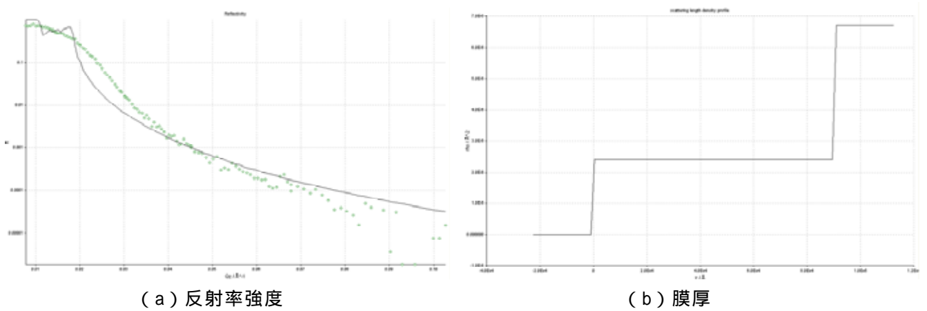
図 6 PVD 処理の TiC 皮膜
