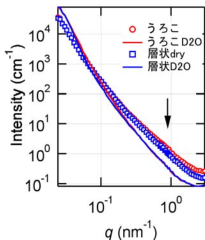
図1 実さび粉末試料（うろこさび、層状さび）の中性子散乱スペクトル
