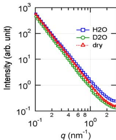
図2 実さび採取まま試料（層状さび、塊状）の中性子散乱スペクトル
